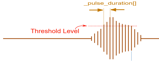
Figure 22. AADD Parameter Visualization
