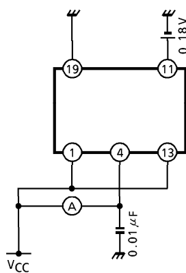
I_{CCQ}
