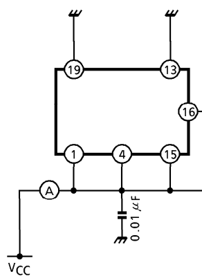
I_{CCO}
