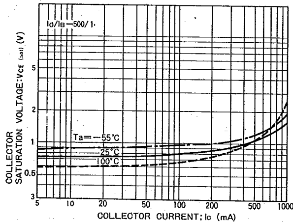
Fig. 40 コレクタ・エミッタ飽和電圧—コレクタ電流特性
