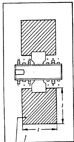
Kupferfläche 35 \mu\text{m} dick Copper area 35 \mu\text{m} thickness
