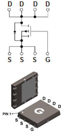
PDFN5×6-8L
