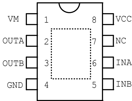
(ESOP-8) TC2466AE
