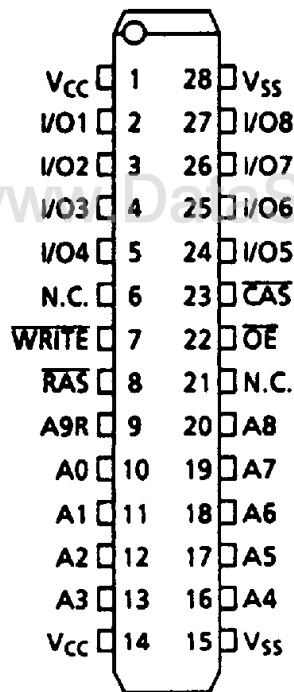
Plastic SOJ
