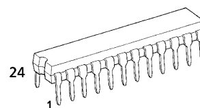
P (DIP24-P-300-2.54) Weight : 1.50g (Typ.)
