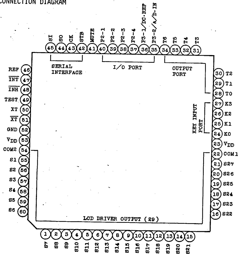
TOP VIEW MINI FP-60PIN
