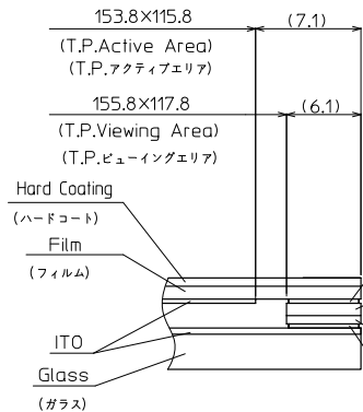
SECTION D-D(NTS)
