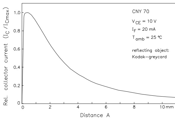
b) CNY 70
