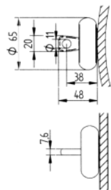
Y部放大 细级分接选择器端子
