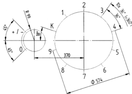
10个触头的布置 (俯视图)
