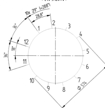
12个触头的引出端子位置 (俯视图)
