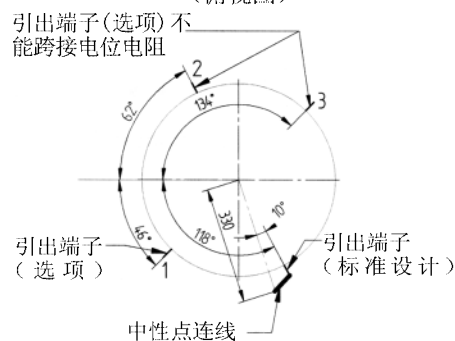
12个触头的布置 (俯视图)
