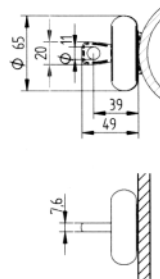
X部放大 转换选择器端子
