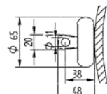
Y部放大 细级分接选择器端子
