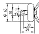
X部放大 转换选择器端子
