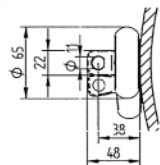
Z部放大 引出端子
