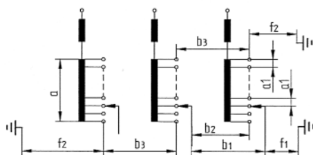
不带转换选择器
