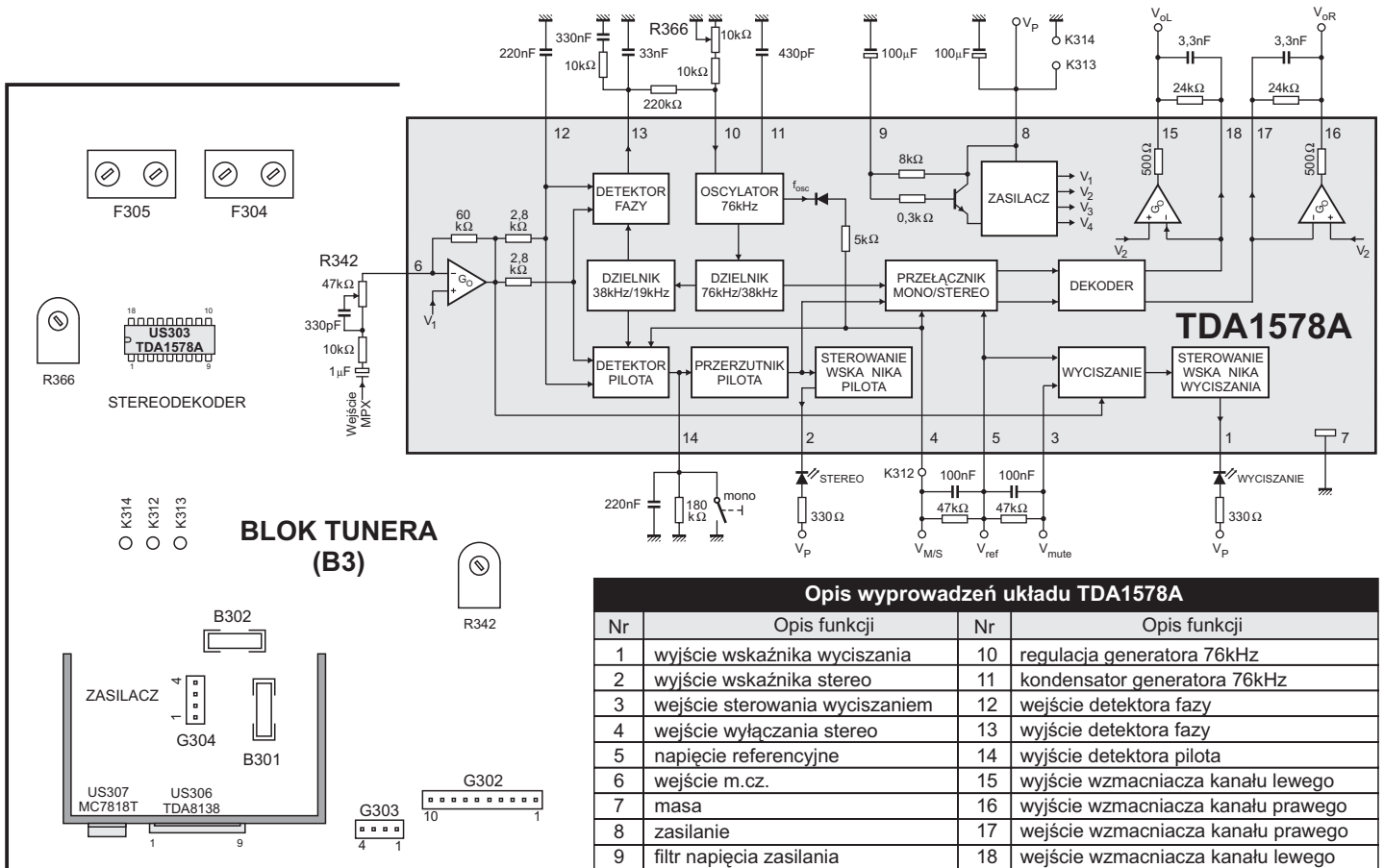
Rys.19. Schemat blokowy układu dekodera stereo TDA1578A ze schematem i opisem wyprowadzeń oraz rozmieszczenie punktów pomiarowych, elementów strojenia i regulacji na bloku tunera B3.
