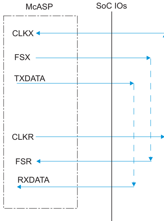
Figure 5-55. McASP1-8 CIOFOI – ASYNC Mode
