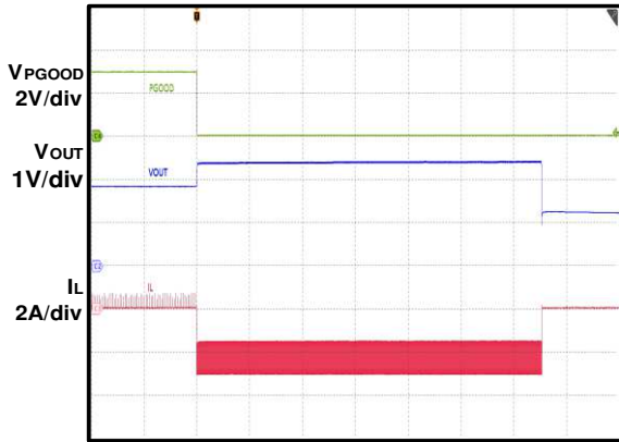
Over-Voltage Protection DEM
