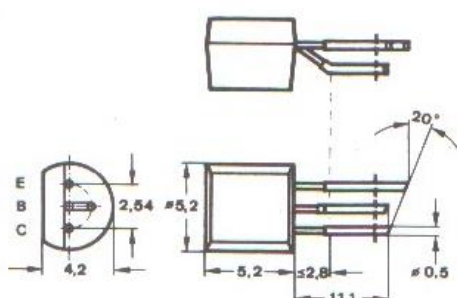
Fig. 3: 10 A 3 DIN 41 868 JEDEC TO 92; Z
