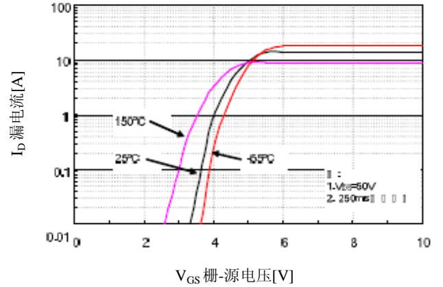
图 2、传输特性
