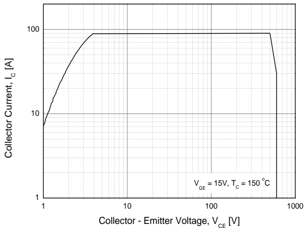
Fig. 15 RBSOA
