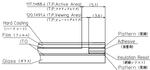
SECTION D-D(NTS)
