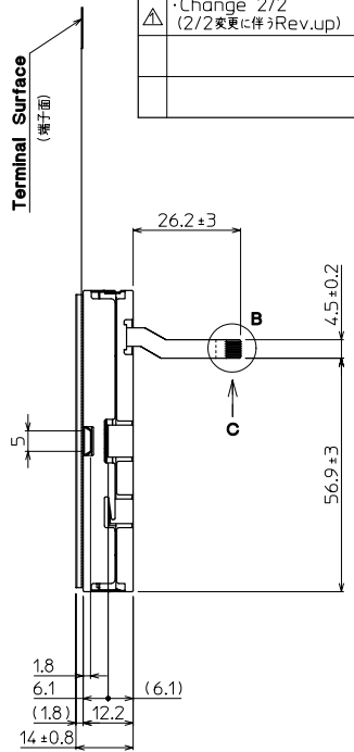
FPC Terminal Layout (FPC 端子レイアウト)
