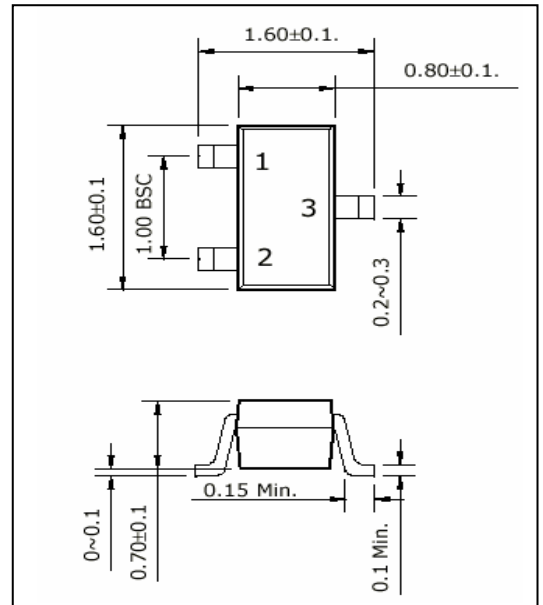
SOT-523
