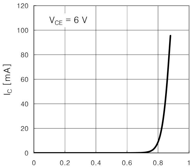
I_C vs. V_{BE}
