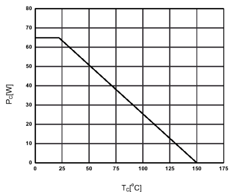
P_C - T_C
