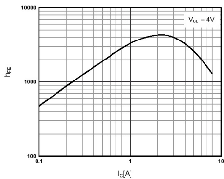
h_{FE} - I_C
