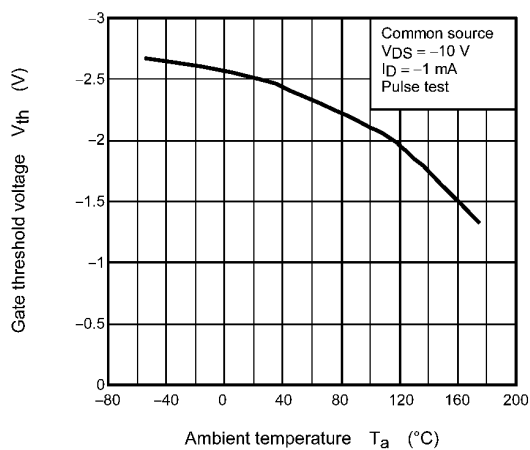
Fig. 9.9 V_{th} - T_a
