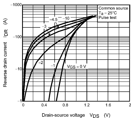
Fig. 9.7 I_{DR} - V_{DS}
