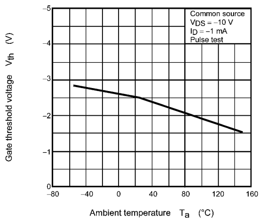
Fig. 9.9 V_{th} - T_a
