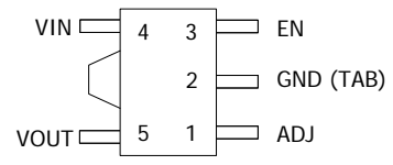
SOT-89-5L
