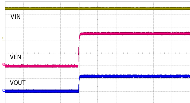
VIN : 1.0V/div, VEN : 1.0V/div, VOUT : 1.0V/div, Time : 5ms/div
