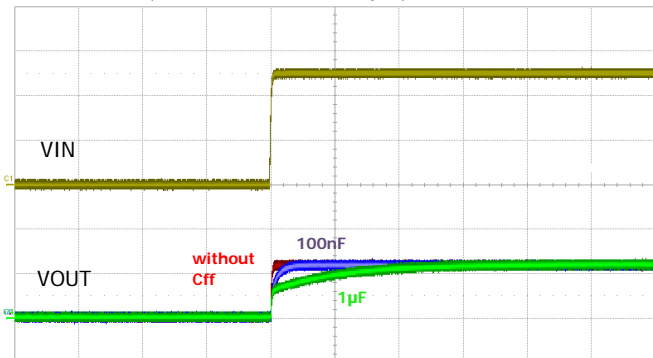
VIN : 1.0V/div, VOUT : 1.0V/div, Time : 10ms/div
