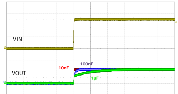
VIN : 1.0V/div, VOUT : 1.0V/div, Time : 10ms/div
