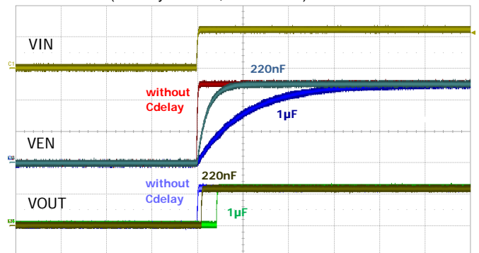
VIN : 2.0V/div, VEN : 1.0V/div, VOUT : 1.0V/div, Time : 10ms/div
