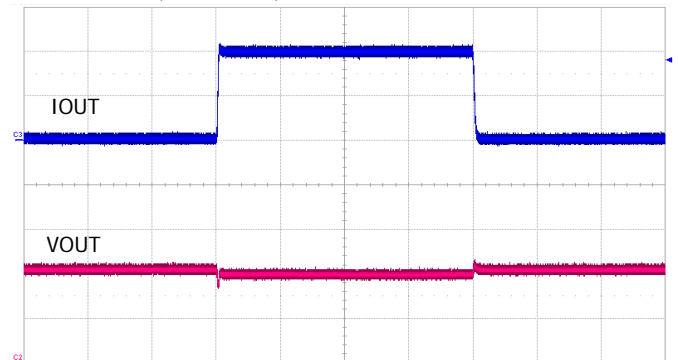
IOUT : 1.0A/div, VOUT : 100mV/div, Time : 500µs/div
