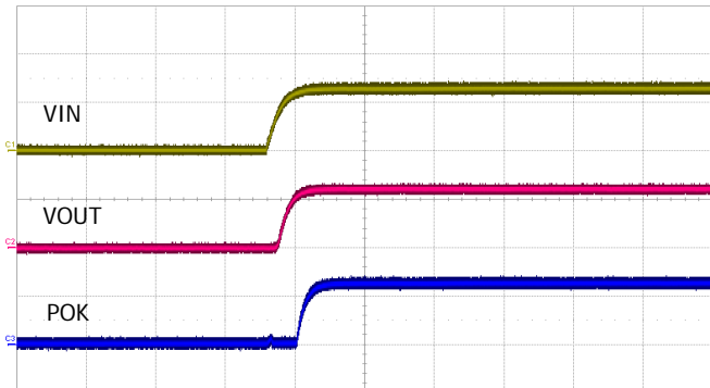
VIN : 2.0V/div, VOUT : 1.0V/div, POK : 2.0V/div, Time : 1ms/div
