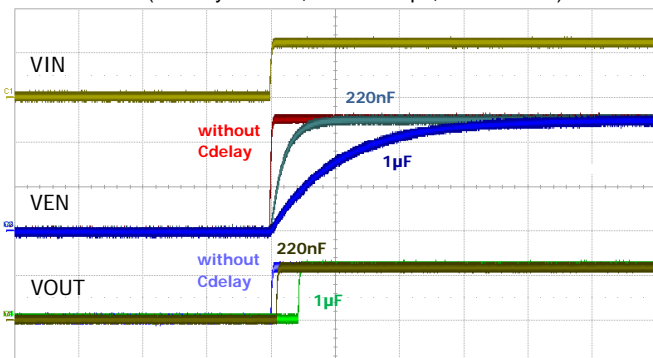
VIN : 2.0V/div, VEN : 1.0V/div, VOUT : 1.0V/div, Time : 10ms/div
