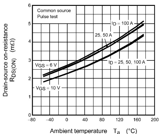
Fig. 9.6 R_{DS(ON)} - T_a
