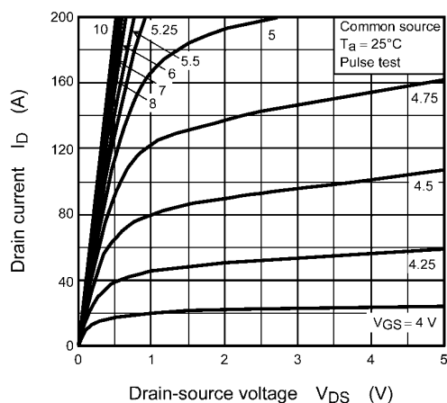
Fig. 9.2 I_D - V_{DS}
