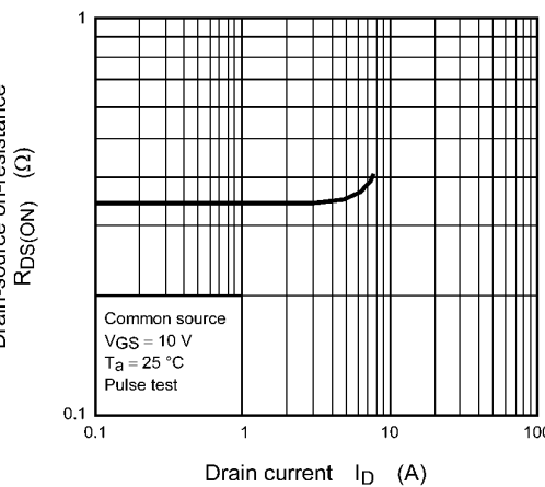
Fig. 8.6 R_{DS(ON)} - I_D
