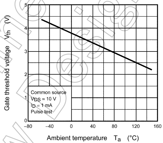
Fig. 8.10 V_{th} - T_a
