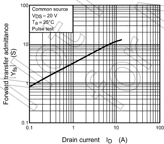
Fig. 8.5 |Y_{fs}| - I_D
