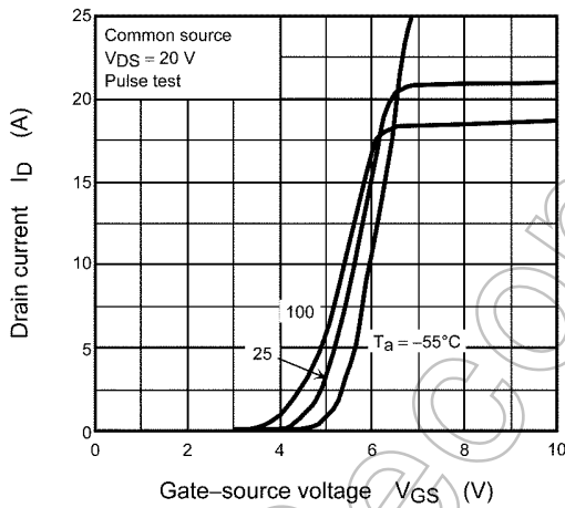
Fig. 8.3 I_D - V_{GS}
