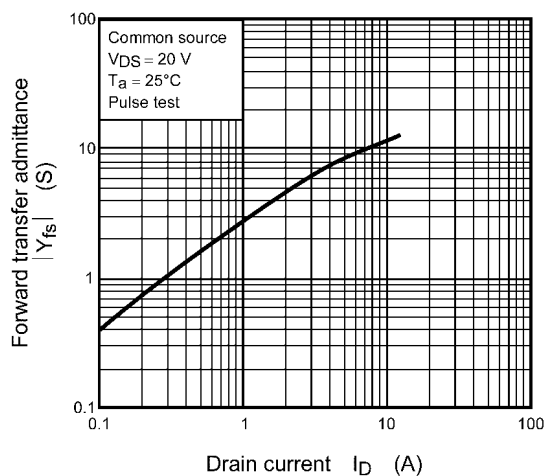
Fig. 8.5 |Y_{fs}| - I_D
