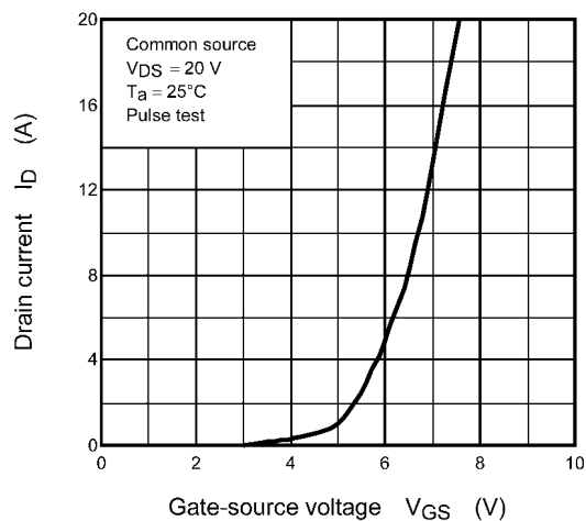
Fig. 8.3 I_D - V_{GS}
