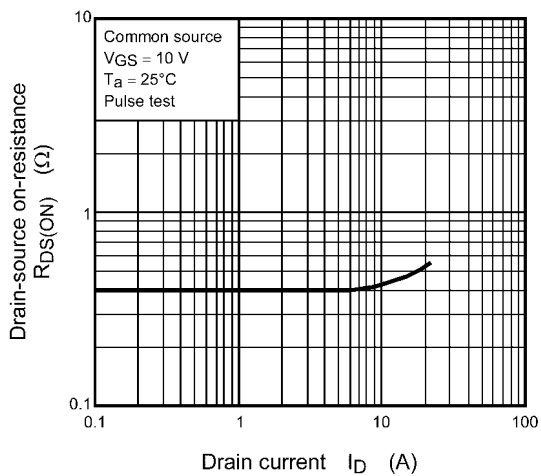
Fig. 8.6 R_{DS(ON)} - I_D
