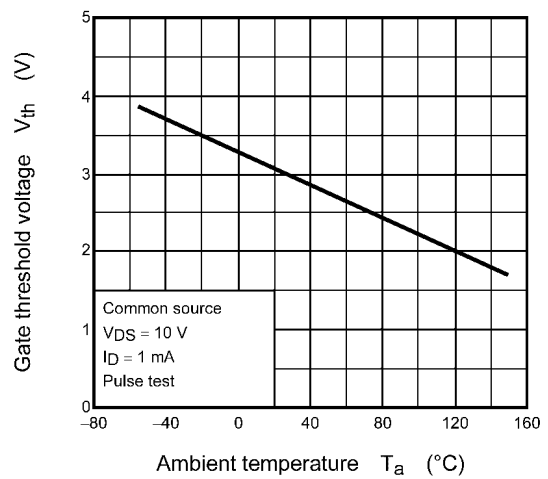
Fig. 8.10 V_{th} - T_a
