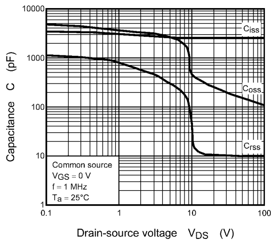
Fig. 8.9 C - V_{DS}
