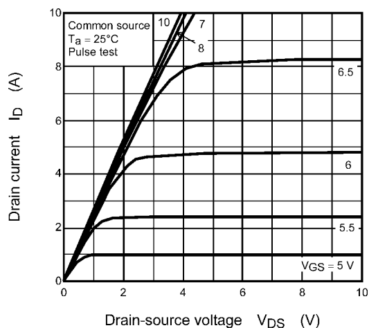
Fig. 8.1 I_D - V_{DS}
