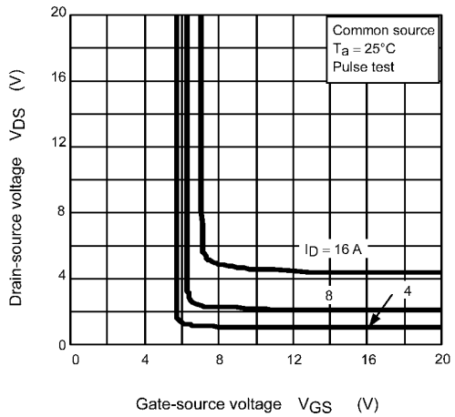
Fig. 8.4 V_{DS} - V_{GS}
