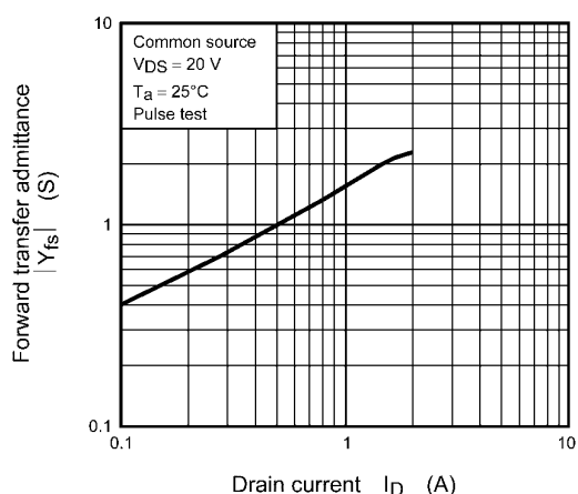
Fig. 8.5 |Y_{fs}| - I_D
