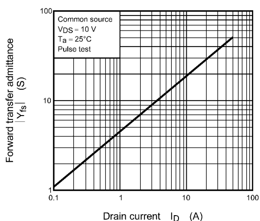
Fig. 8.5 |Y_{fs}| - I_D
