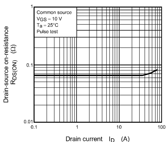
Fig. 8.6 R_{DS(ON)} - I_D
