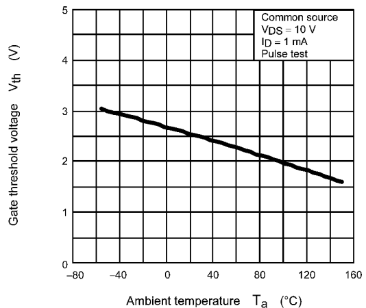
Fig. 8.10 V th - T a
