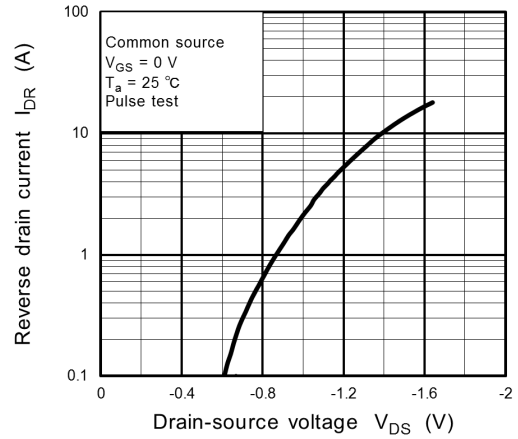
Fig. 8.8 I_{DR} - V_{DS}
