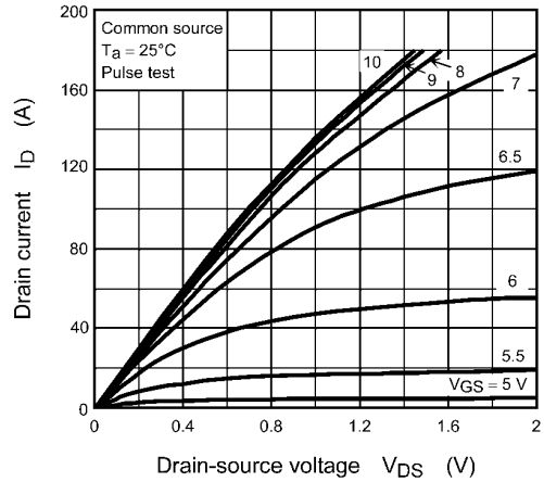
Fig. 9.2 I_D - V_{DS}
