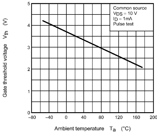
Fig. 8.9 V_{th} - T_a
