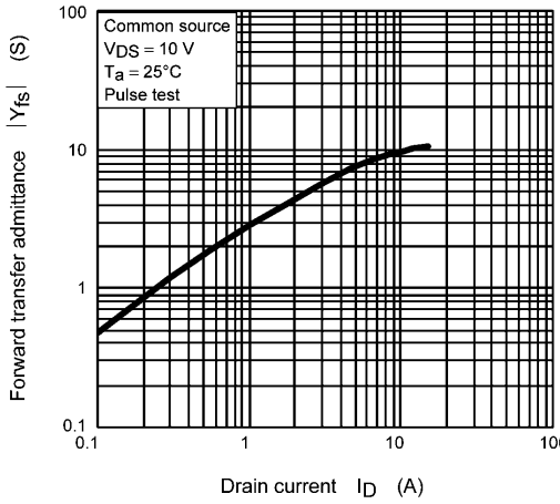
Fig. 8.5 |Y_{fs}| - I_D
