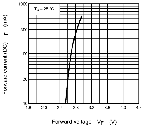
Fig. 8.1 I_F - V_F
