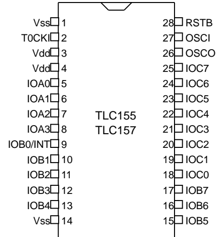
SSOP
