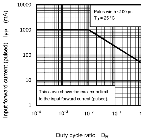
Fig. 11.3 I_{FP} - D_R
