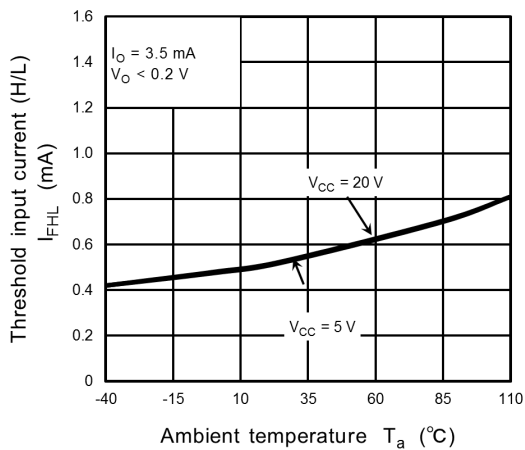
Fig. 13.2.2 I_{FHL} - T_a
