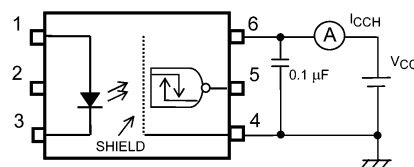
Fig. 13.1.4 I_{CCH} Test Circuit
