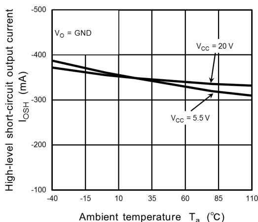
Fig. 13.2.10 I_{OH} - T_a
