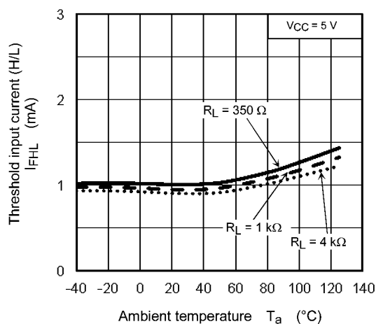
Fig. 12.2.7 I_{FHL} - T_a
