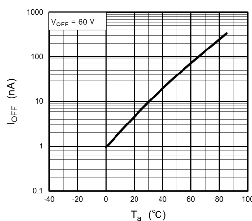
Fig. 12.1.10 I_{OFF} - T_a
