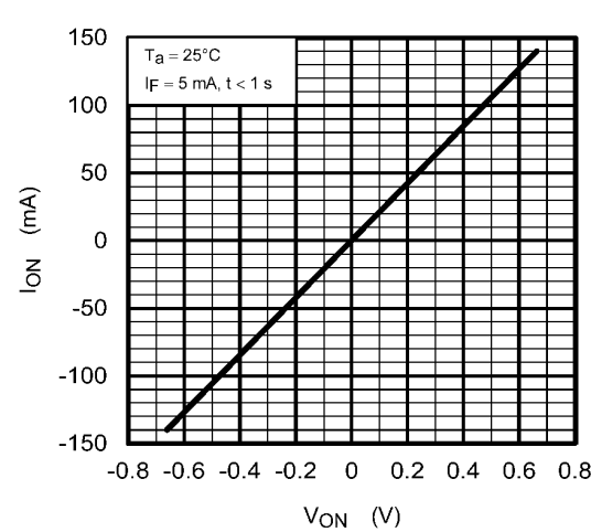
Fig. 12.4 I_{ON} - V_{ON}
