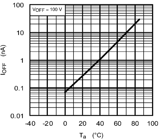
Fig. 12.1.9 I_{OFF} - T_a
