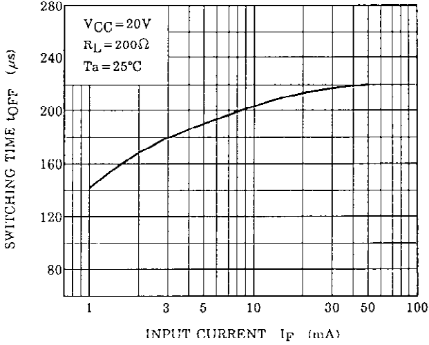
t_{OFF} - I_F
