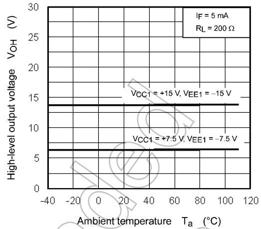
Fig. 12.2.8 V_{OH} - T_a
