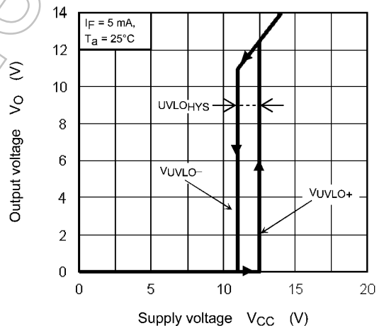
Fig. 12.2.12 V_O(V_{UVLO}) - V_{CC}
