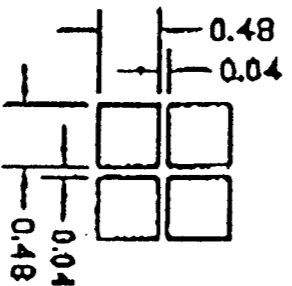
DETAIL A1
